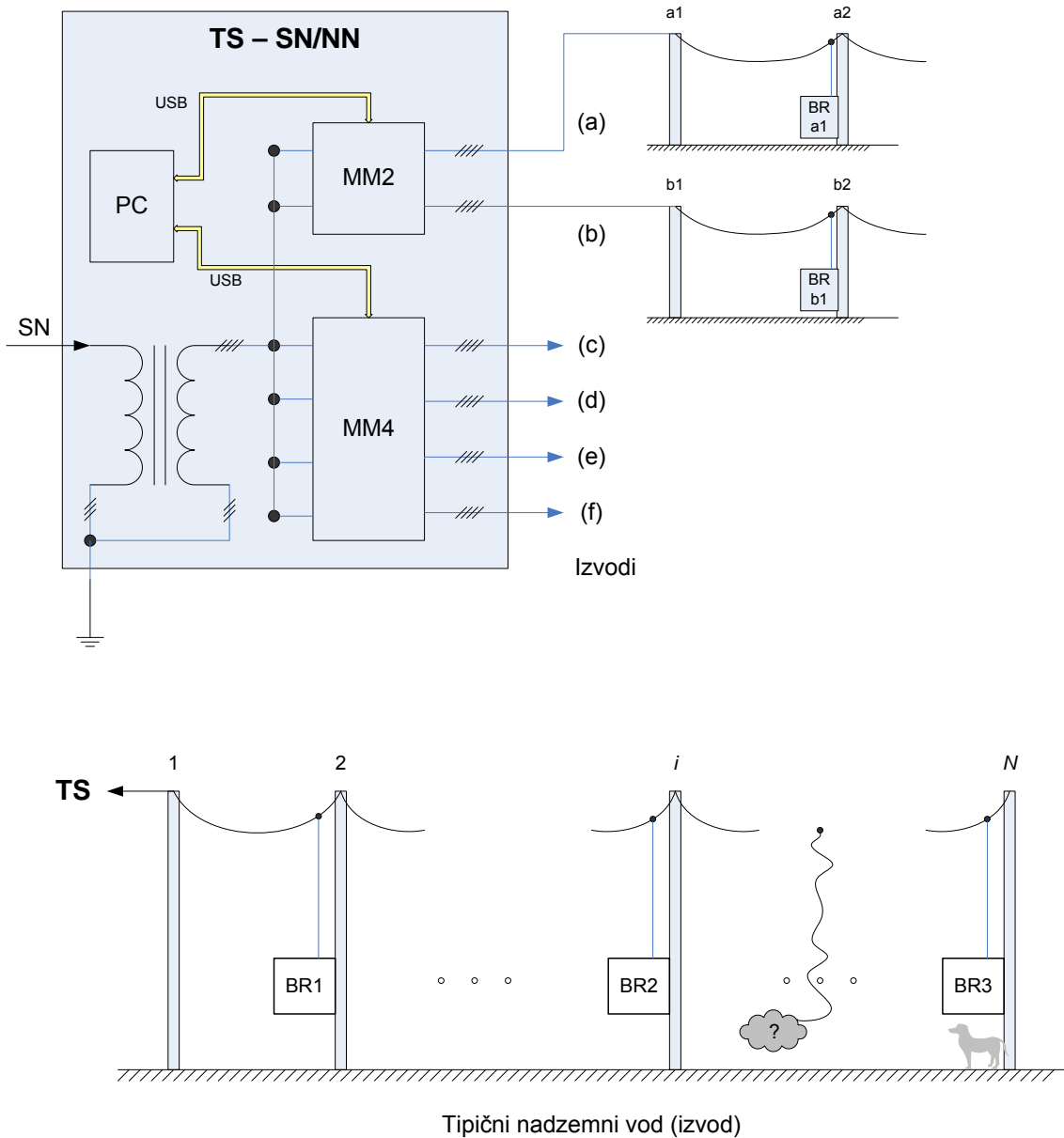
Slika 1. Skica sistema u kom se primenjuje postupak: a) prikaz dela sistema u trafostanici; b) prikaz dela sistema na vodu
