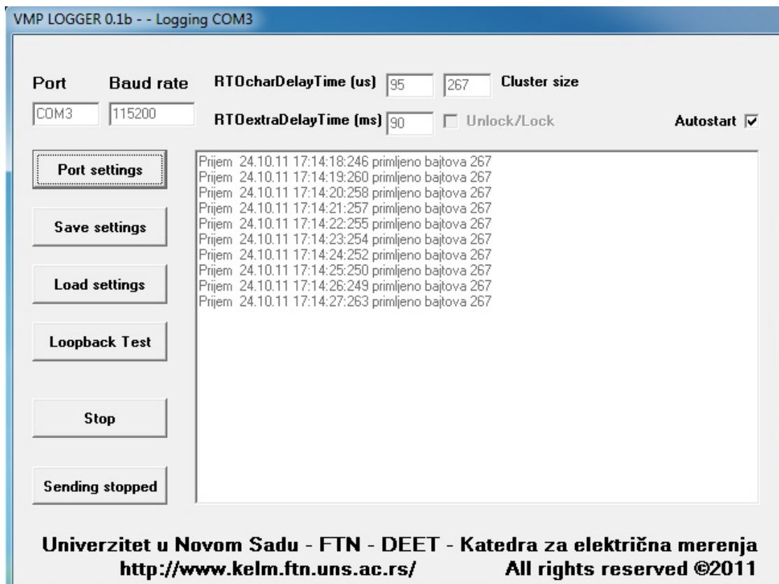
Slika 3. Prikaz kontrole priključenja analizatora snage
